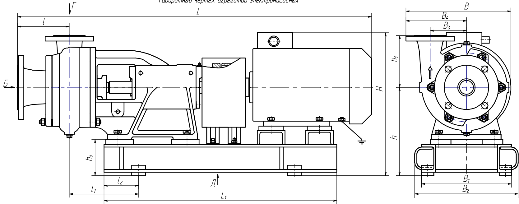
Продолжение приложения Б Габаритный чертеж агрегатов электронасосных
